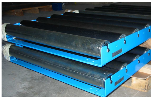
Convoyeurs à rouleaux libres équipés de l'option rouleaux moteurs renforcés
